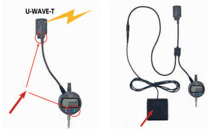
Câble sans connexion pédale de validation
